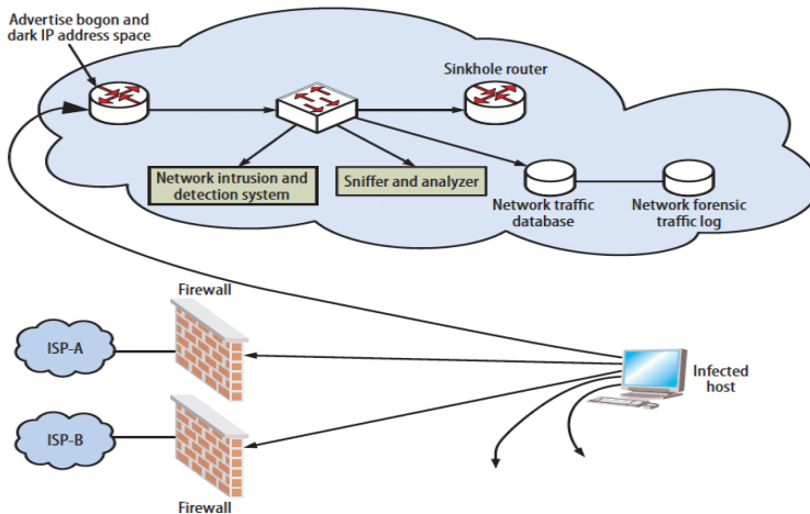
Рисунок 1 – Методологія розслідування мережесих атак
