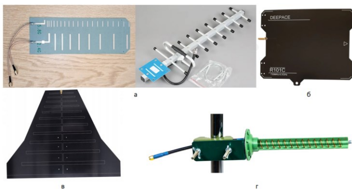
а – YAGI антени; б – антена Вівальді; в – логоперіодична антена; г – спіральна антена. Рисунок 1 – Направлені антени.
