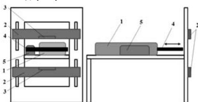
Рис. 1. Эскиз стенда для динамических испытаний ГКС
