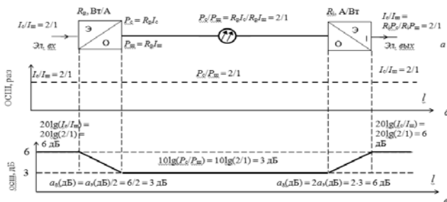
Рисунок 3 – Схема оптического ЛТ а и диаграммы изменения ОСШ (раз) б и осш (дБ) в для идеального тракта без собственных шумов для случая, когда на входе I_c/I_{ш} = 2/1
