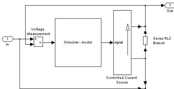
Рис. 2. Общая схема блока нелинейного резистора
