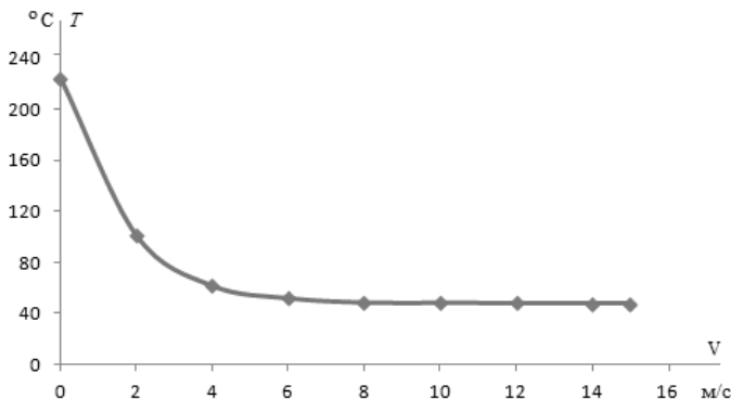
Рис. 2. Вплив швидкості повітряного потоку в каналі системи охолодження на тепловий режим модулів
