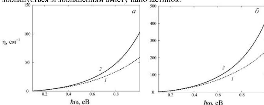
Рис. 1. Частотні залежності \eta(\omega) нанокompозиту із частинками Au в KCl при \beta = 0,004 (а) та \beta = 0,016 (б): 1 – \epsilon_\infty = 1 , m^* = m_e ; 2 – \epsilon_\infty = 9,84 , m^* = 1,32m_e .
