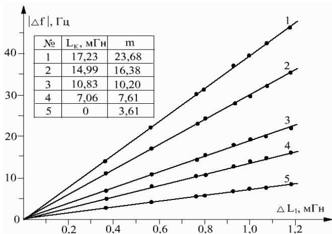
Рис. 2. Приращение частоты \Delta f генератора как функция индуктивности датчика L_1 для разных значений компенсирующей индуктивности L_K
