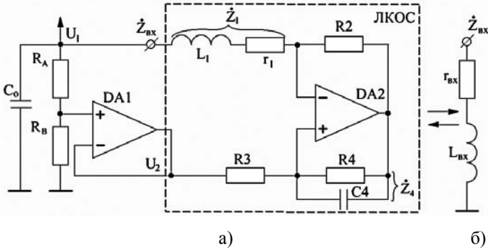
Рис. 1. Измерительный генератор (а) и эквивалентное представление ЛКОС (б)
