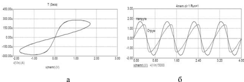
Рис. 2. Характеристики мемристора: а – статичні ; б – динамічні
