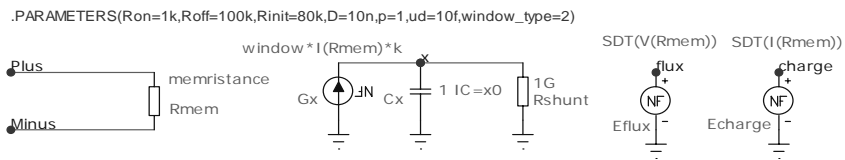
Рис. 1. Схема заміщення моделі мемристора
