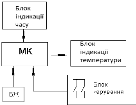
Рис. 1. Структурна схема світлодіодного годинника
