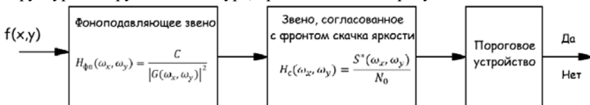
Рис. 2. Структура обнаружителя начальной точки контура изображения
