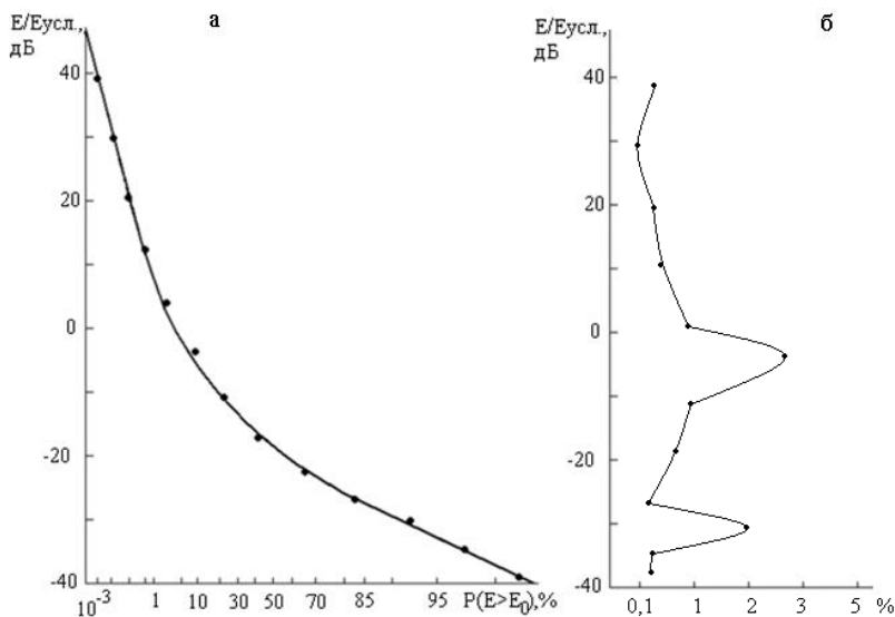
Рис. 1. Сравнение экспериментальных (точки) и теоретических (сплошная линия) из отчета МККР № 322 значений функции распределения амплитуд (а) и их погрешности (б)
