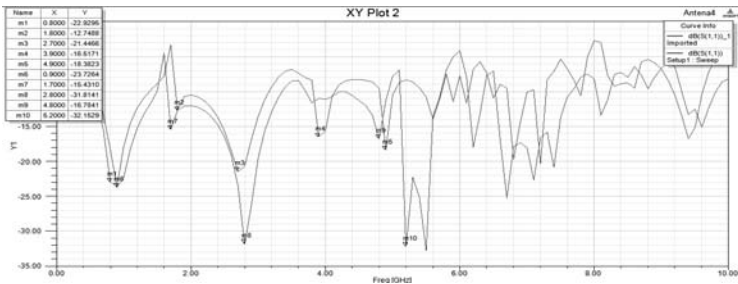
Рис. 3. Частотные характеристики антенны с DNG и ENG- метаматериалами
