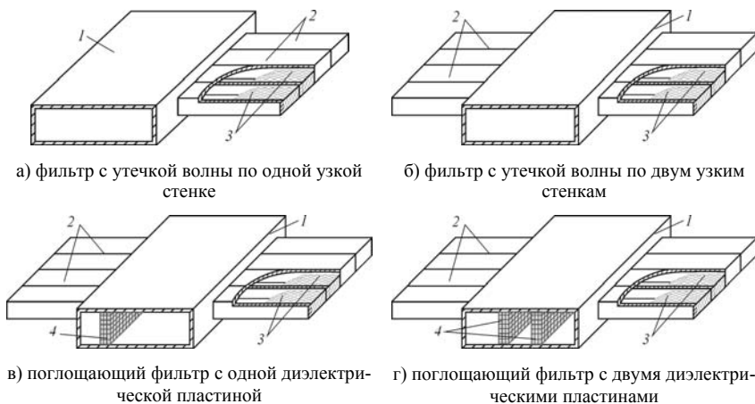
Рис. 1. Разновидности конструкций поглощающего фильтра гармоник: 1 – основной волновод; 2 – боковые волноводы; 3 – поглощающая нагрузка; 4 – диэлектрическая пластина
