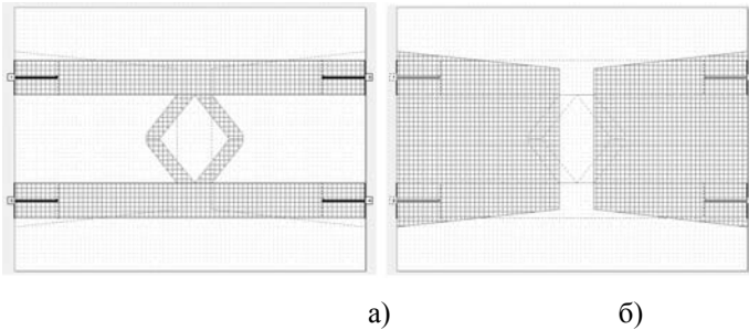
Рис. 4. Топология НО в системе MWO: а) МПЛ структура, б) ЦЛ структура
