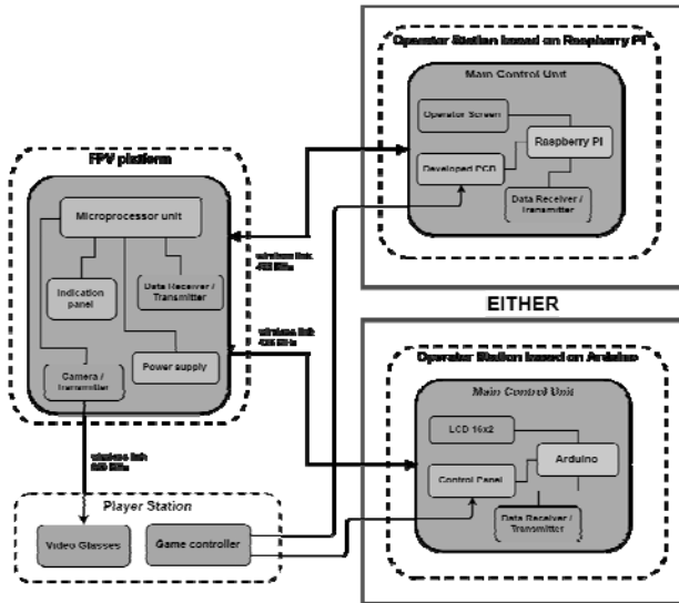
Рис. 1. Архітектура системи
