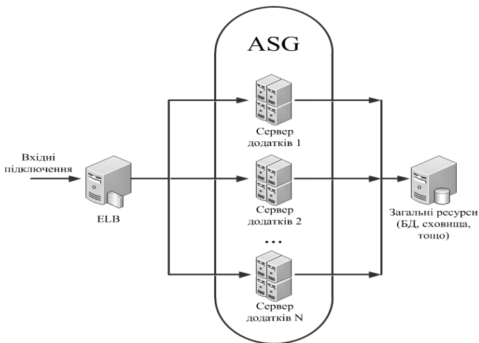
Рис. 1. Модель системи
