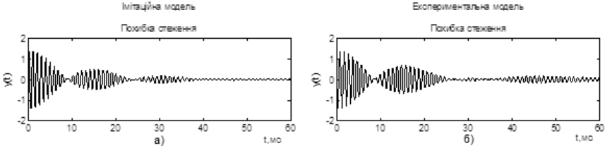
Рис. 1. Результати дослідження імітаційної (а) та експериментальної (б) моделей для випадку \Delta f = 20 Гц ( f_{вх} = 1020 Гц) і \Delta\varphi = 0^\circ .
