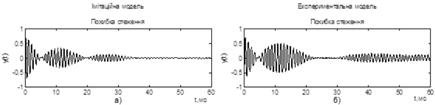
Рис.2. Результати дослідження імітаційної (а) та експериментальної моделі (б) для випадку \Delta f = -5 Гц ( f_{вх} = 995 Гц) і \Delta\varphi = 45^\circ .
