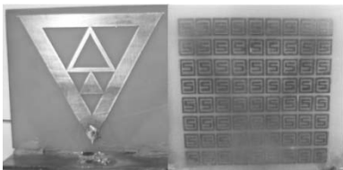
Рис. 1. Геометрия модифицированной салфетки Серпинского
