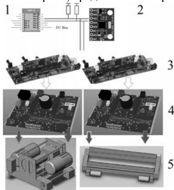
Рис. 1. Общая структура встраиваемой системы с использованием беспроводного модуля ESP8266
