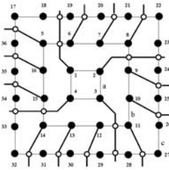
Рис. 1. Фрагмент корпуса на 36 выводов и проведение соединений.
