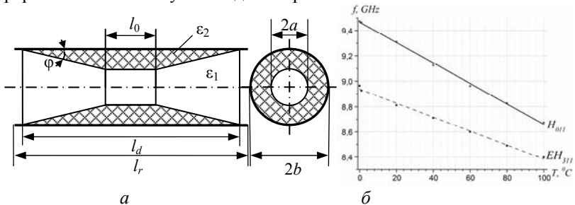
Рис. 1. Відкритий хвильовідний резонатор (а);
