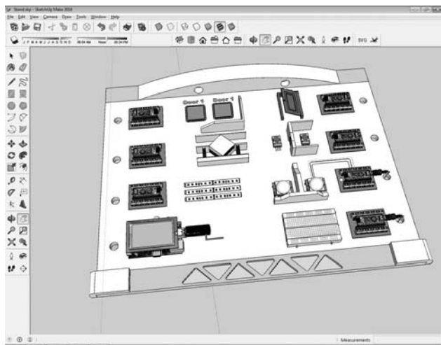
Рис. 1. Трехмерная модель проектируемой платформы
