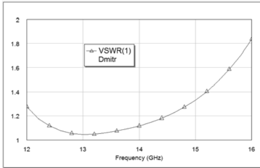
Рис. 6. КСВ ответвителя в диапазоне частот
