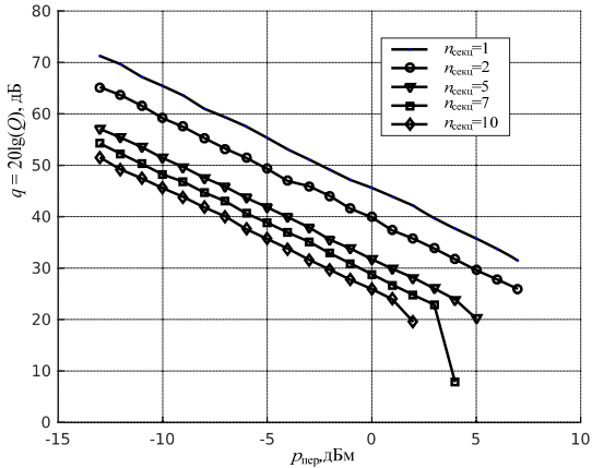
Рис. 1. Показатели качества канала ВОСП ( \alpha = 0,2 дБ/км; D=16,75 пс/нм/км); \gamma = 1,31 1/Вт/км; L_{секц}=100 км; n_f=4 дБ)
