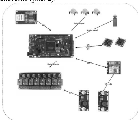
Рис. 2. Архитектура прототипа
