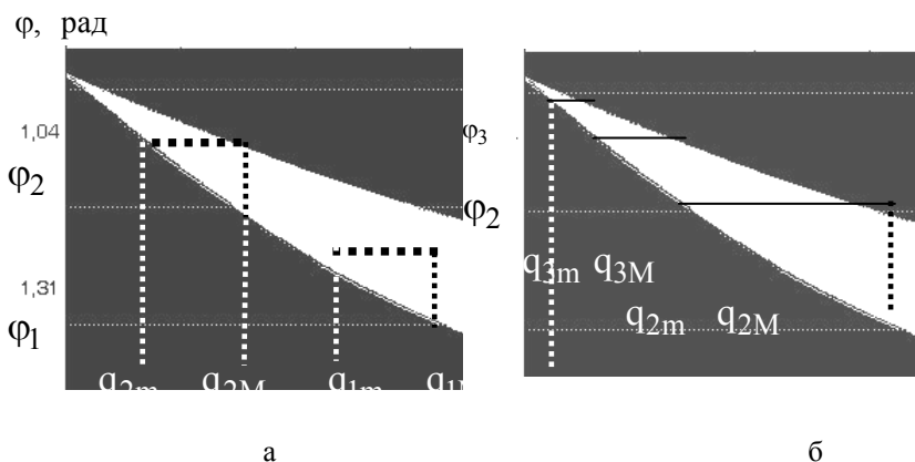
Рис. 2. Розподіл відносної похибки визначення вертикальної похідної I_a \delta q(\varphi, q) (а). Приклад неперервного діапазону реконструкції (б)
