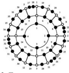
Рис. 2. Топологическая модель корпуса на 36 выводов и проведение соединений.
