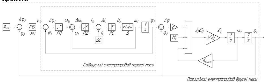
Рисунок 1 - Функціональна схема слідкуючого приводу, де РП - регулятор положення; РШ - регулятор швидкості; РС - регулятор струму; СК - силовий комутатор; Д - модель двигуна
