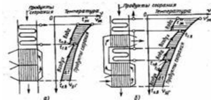
Рисунок 1 - Схеми одноступінчастої та двоступінчастої компоновки (для Е-75-40ГМ)
