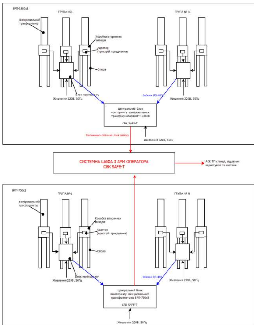
Рисунок 1 – Структура системи
